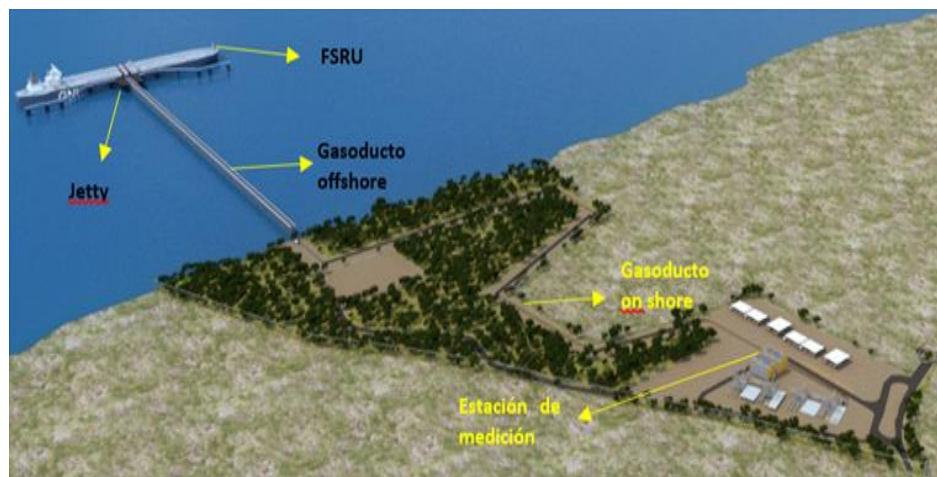
Figura 2 Maqueta proyecto
