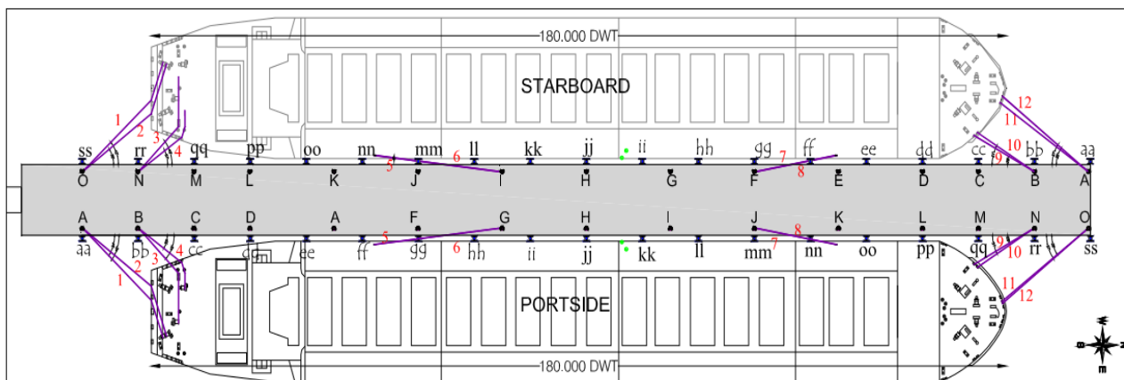
Ilustración 1: Distribución de amarres y defensas. Muelle Puerto Brisa
